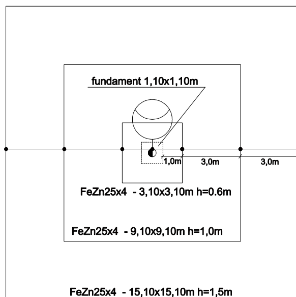
maszty nr 6-9
